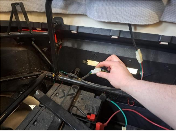
Avaa oikeapuolen takavalon liitin.
