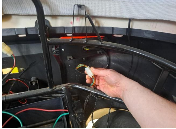
Avaa vasemman takavalon liitin.
