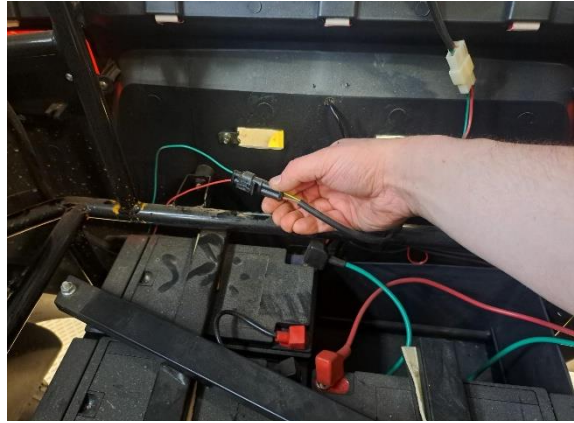
Avaa peruutusvalon liitin.
